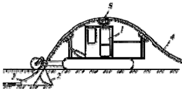
Рисунок 8 - Ножевой трубнозаглубитель
