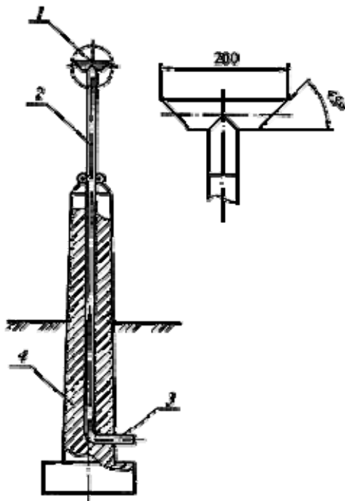
1 - оголовок; 2 - вытяжная труба; 3 - отводная труба; 4 - фундамент
