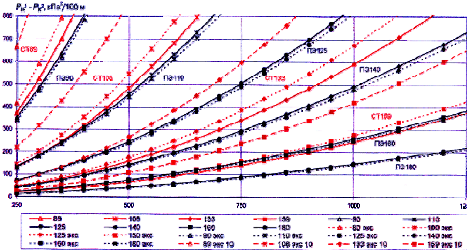
Удельные потери давления для стальных и полиэтиленовых труб (новых и бывших в эксплуатации) низкого давления ( Q = 250-1250 \text{ м}^3/\text{ч} , \rho = 0,73 \text{ кг/м}^3 , \gamma = 1,4 \times 10^{-6} \text{ м}^2/\text{с} )
