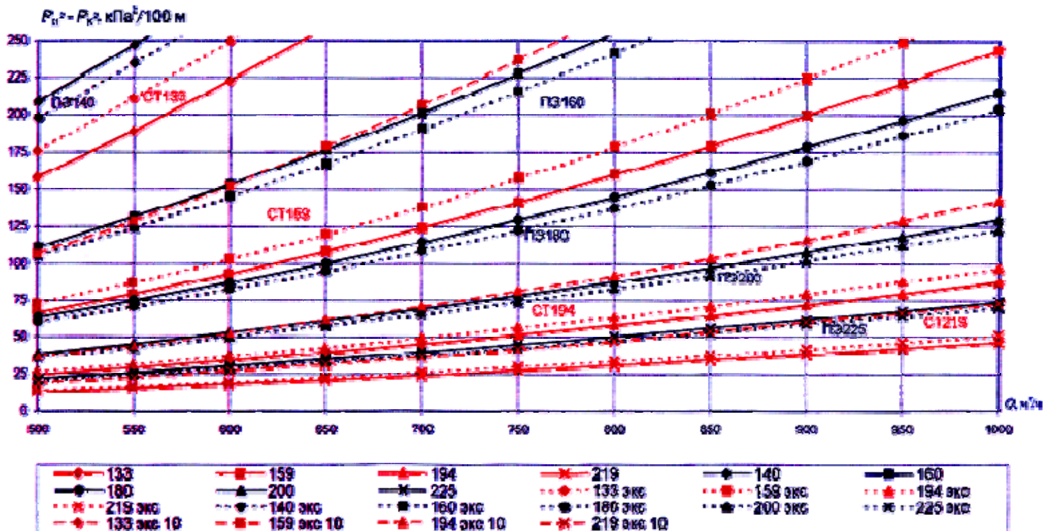
Удельные потери давления для стальных и полиэтиленовых труб (новых и бывших в эксплуатации) высокого давления ( Q 500-1000 м 3 /ч, \rho=0,73 \text{ кг/м}^3 , \nu=1,4 \times 10^{-6} \text{ м}^2/\text{с} )
