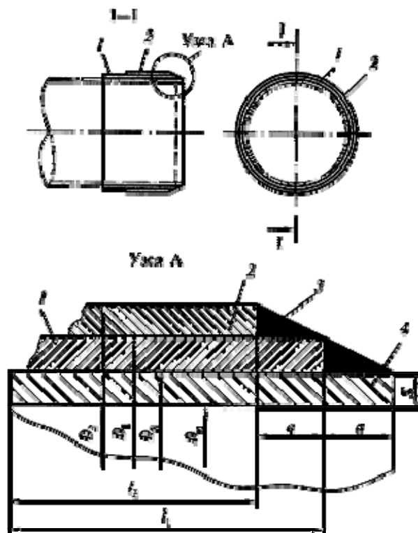
Рисунок 11 - Устройство кольцевого ножа на конце футляра
