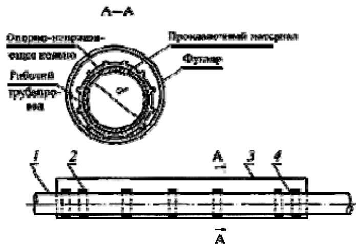
Рисунок 3 - Прокладка газопровода в футляре
