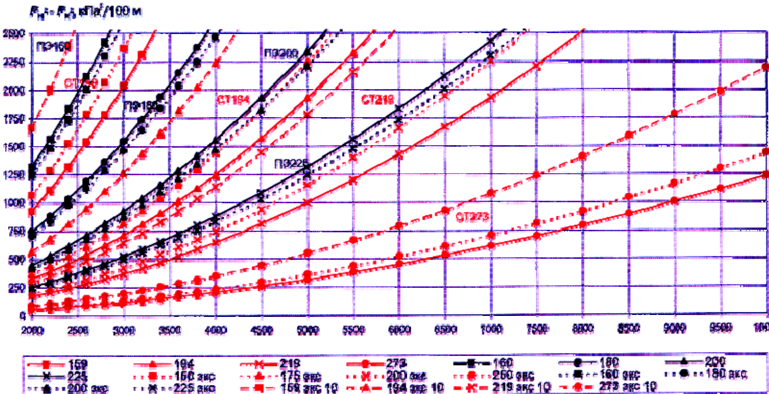
Удельные потери давления для стальных и полиэтиленовых труб (новых и бывших в эксплуатации) высокого давления ( Q 2000-10000 м 3 /ч, \rho=0,73 \text{ кг/м}^3 , \nu=1,4 \times 10^{-6} \text{ м}^2/\text{с} )
